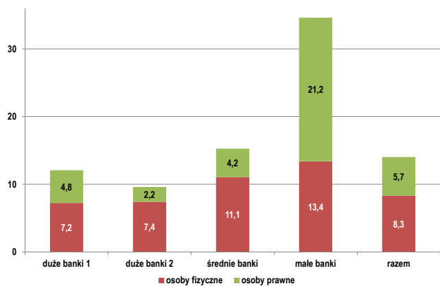
Wykres 2.4 Odsetek funduszu udziałowego przypadającego na członków posiadających 5% lub więcej kwoty funduszu (%) – 30.06.2013 r.
